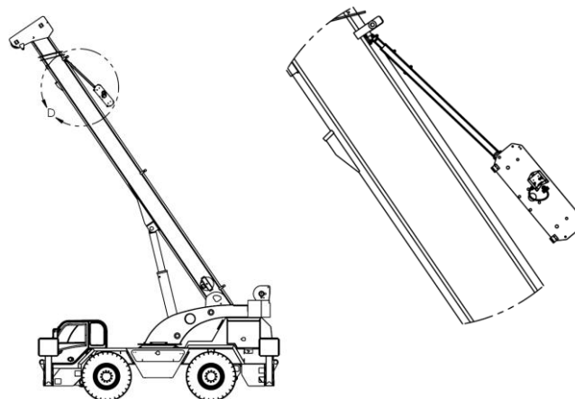
Dibujo: Instalación típica en la pluma principal de una grúa para la medición de la carga y de la longitud de desenrollamiento del cable
